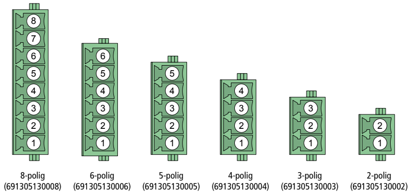
Abb. 9: Würth-Grundleiste (Draufsicht)
