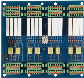
Abb. 4: Relaisboard ADQ-SCU-RB-16/8
