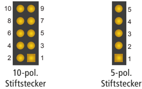
Abb. 10: Stiftstecker (Draufsicht)
