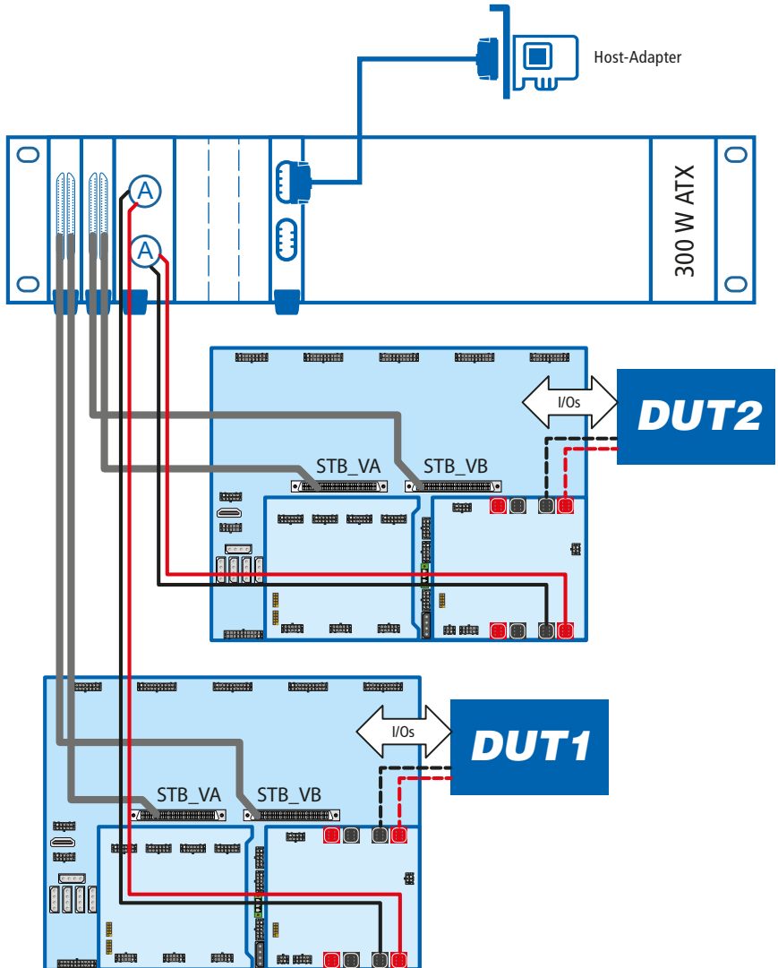
Abb. 7: Beispiel-Systemkonfiguration
