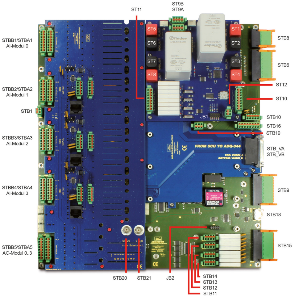
Abb. 8: Steckerpositionierung
