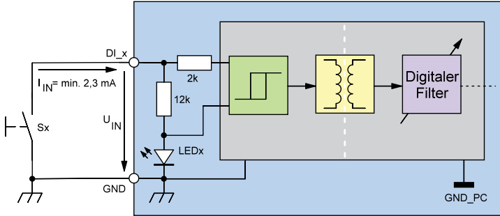
Abb. 3: Beschaltung der isolierten Digital-Eingänge
