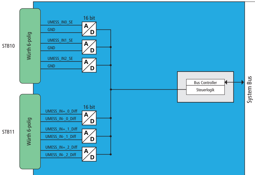
Abb. 10: Blockschaltbild analoge Eingänge
