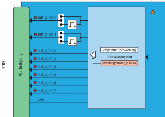
Abb. 4: Digitaler Ausgang im Detail
