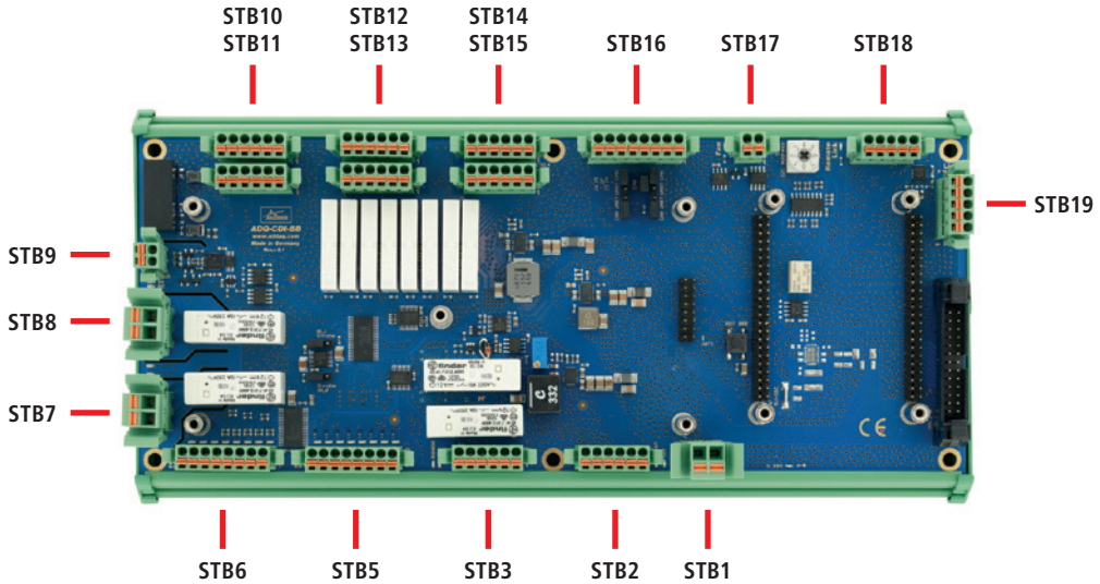
Abb. 16: ADQ-CDI-BB v2 mit Steckerposition
