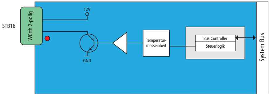
Abb. 11: Blockschaltbild Lüftersteuerung
