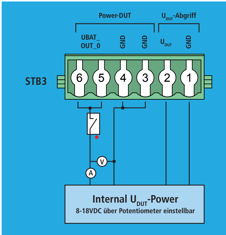
Abb. 6: Blockschaltbild Powermesskanäle
