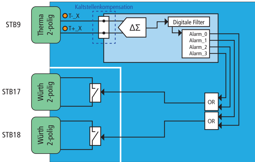
Abb. 7: Blockschaltbild Temperaturmesskanal inkl. Alarm-Relais
