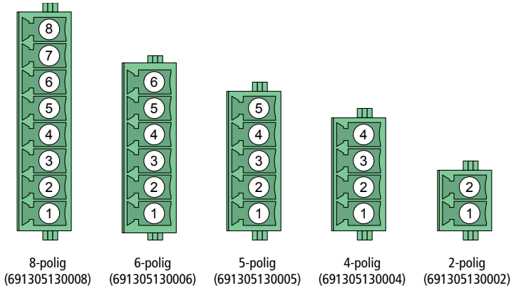
Abb. 17: Würth-Grundleiste Typ WR-TBL 3051 (Draufsicht)
