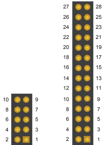
Abb. 19: Stiftstecker, 2,54mm (Draufsicht)
