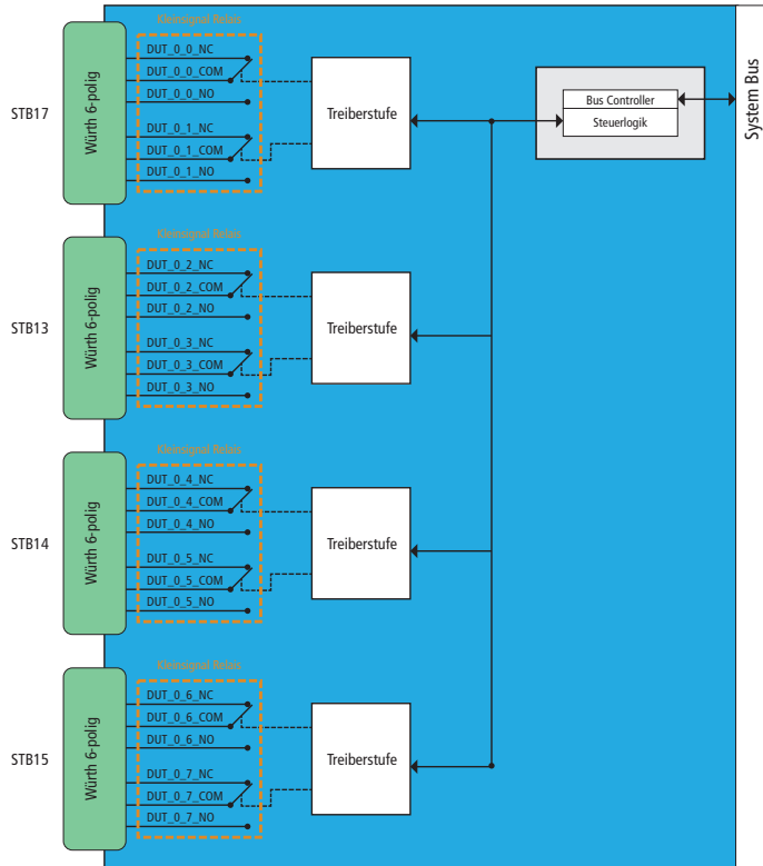
Abb. 9: Blockschaltbild Relais
