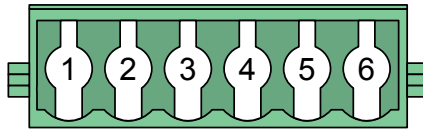
Abb. 29: Würth 691305530006
