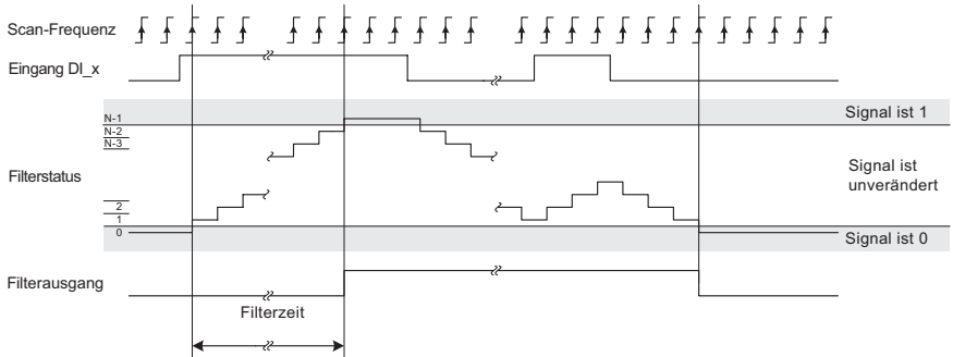
Abb. 2: Digitaler Eingangsfilter
