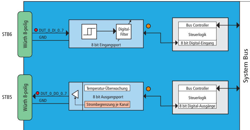
Abb. 1: Blockschaltbild digitale Ein- und Ausgänge
