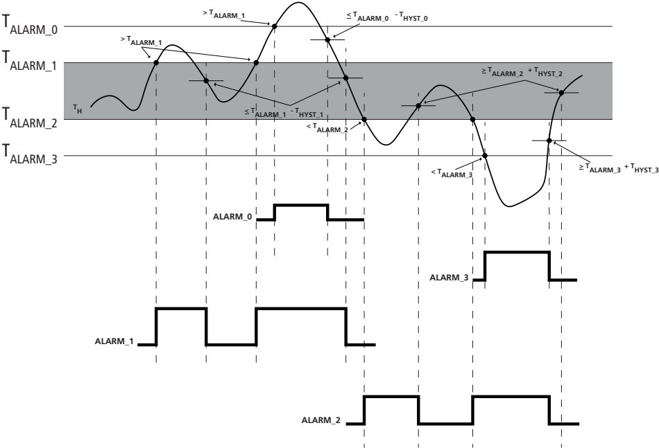
Abb. 8: Alarmschwellwerte
