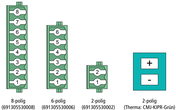
Abb. 18: Therma/Würth-Grundleiste Typ WR-TBL 3055 (Draufsicht)
