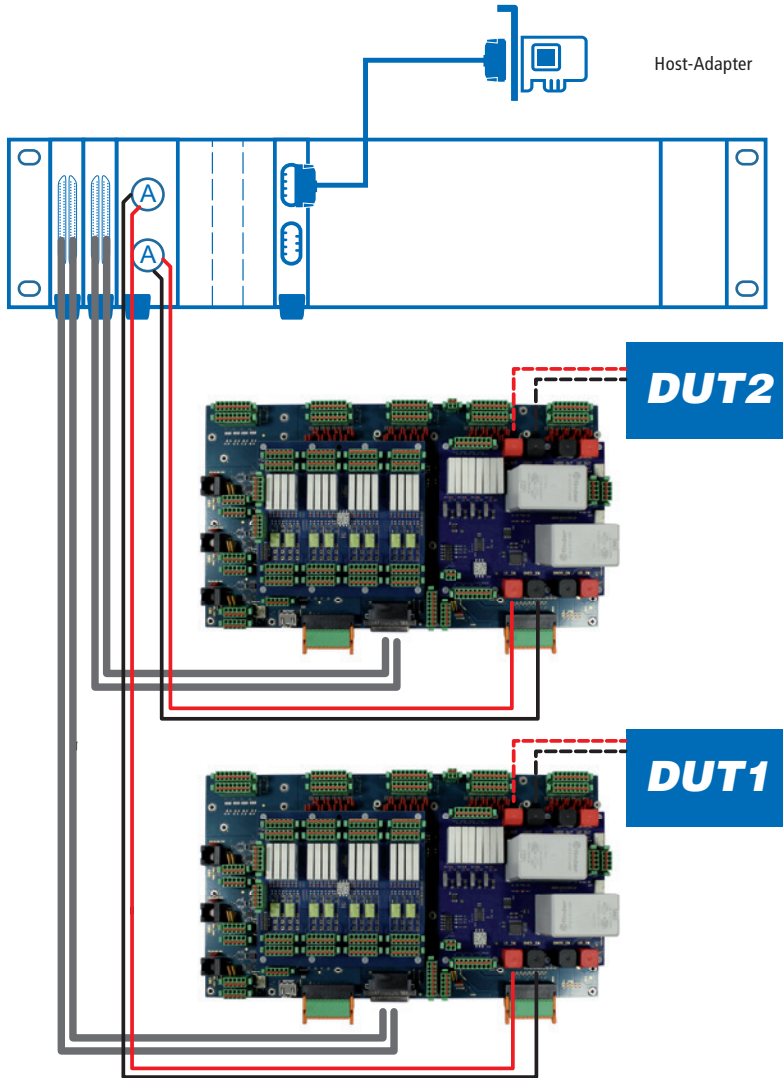
Abb. 6: Beispiel-Systemkonfiguration
