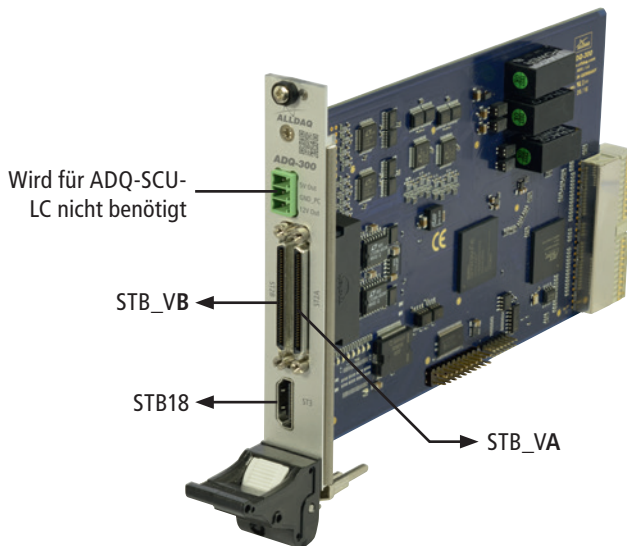
Abb. 5: Multifunktionskarte ADQ-344
