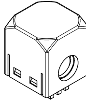
Abb. 22: 8 x einpolige Hochstrom-Steckverbinder vom Typ: Würth Electronic REDCUBE Direct Plug Terminal WP-PLUG.
