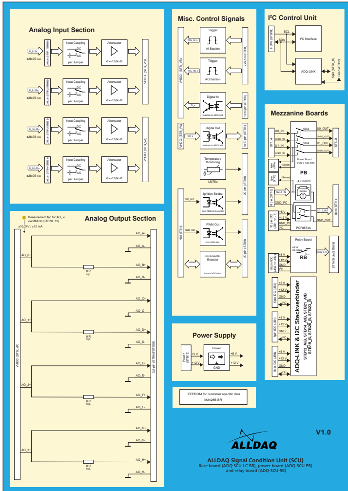
Abb. 1: Blockschaltbild ADQ-SCU-LC
