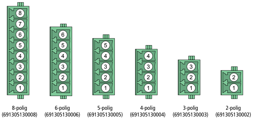
Abb. 8: Würth-Grundleiste (Draufsicht)
