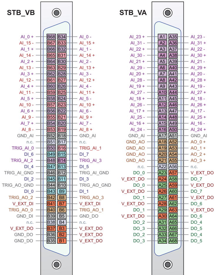
Abb. 20: Anschlussbelegung STB_VA und STB_VB
