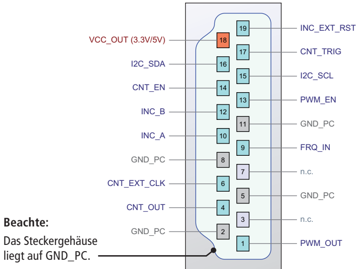
Abb. 18: HDMI-Steckverbinder (STB18)
