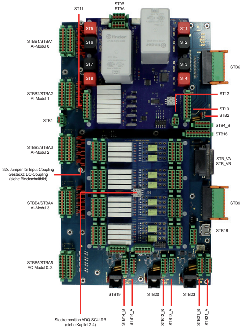
Abb. 7: Steckerpositionierung
