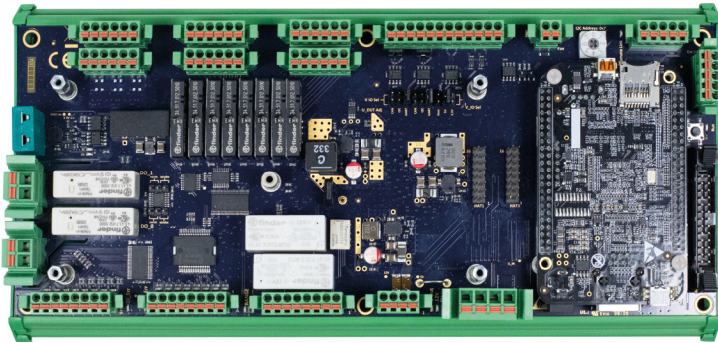
Figure 17: ADQ-CDI-BB mit Beagle Bone Black Einplatinen-Computer
