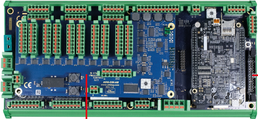
Figure 14: Position Erweiterungsplatten (HATs)
