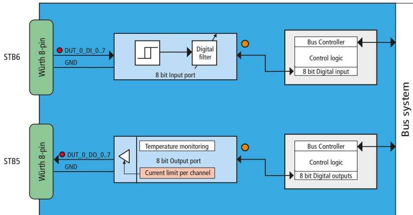
Figure 1: Blockschaltbild digitale Ein- und Ausgänge
