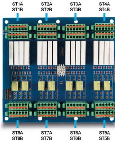
Abb. 4: Relaisboard ADQ-SCU-RB-16/8
