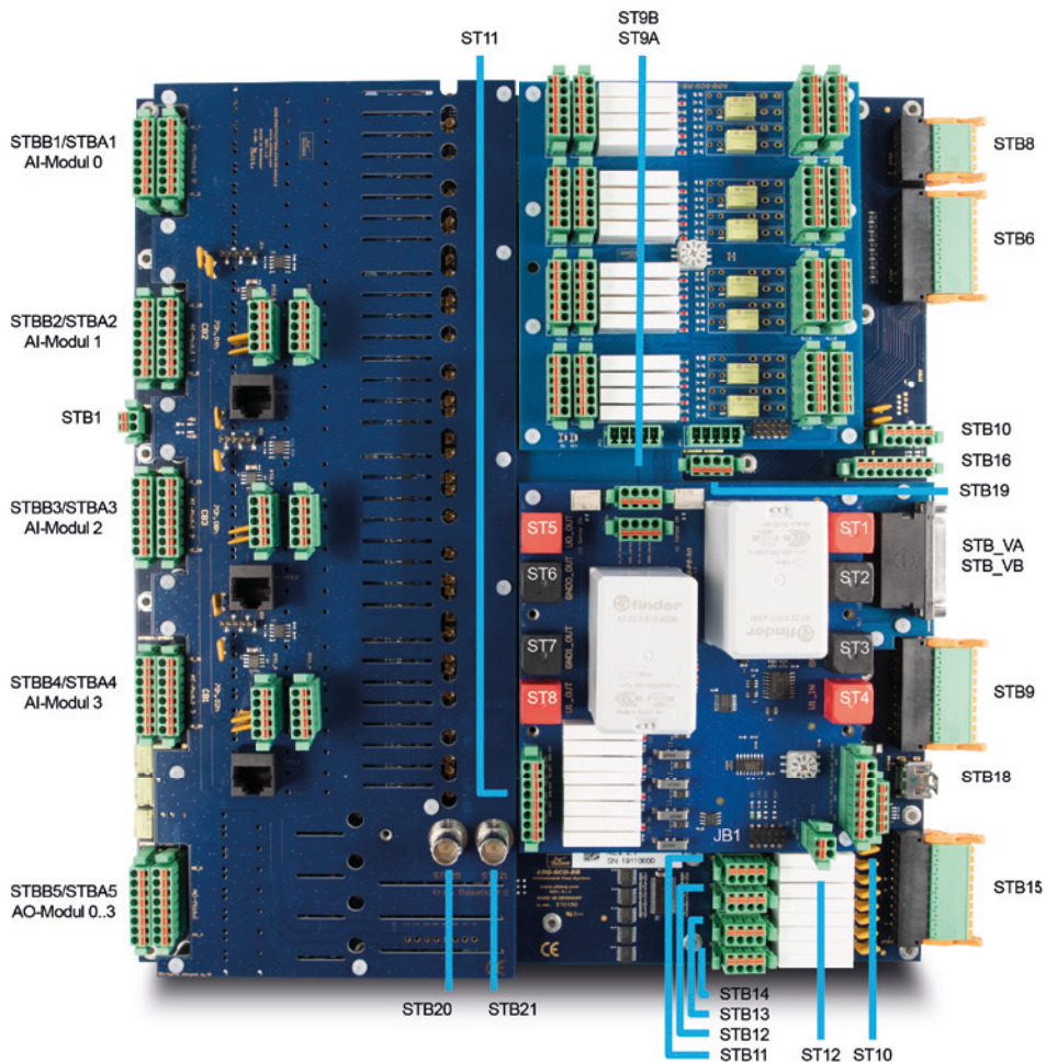
Abb. 8: Steckerpositionierung
