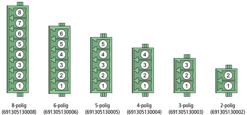
Abb. 9: Würth-Grundleiste (Draufsicht)
