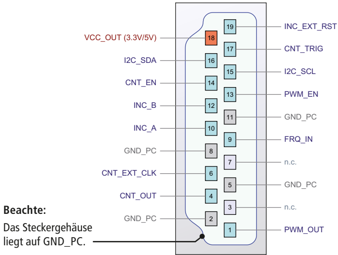
Abb. 23: HDMI-Steckverbinder (STB18)
