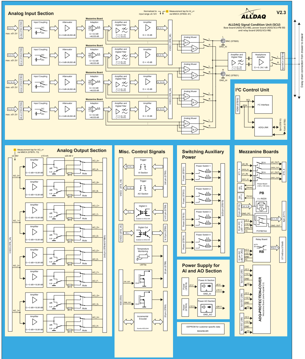
Abb. 1: Blockschaltbild ADQ-SCU
